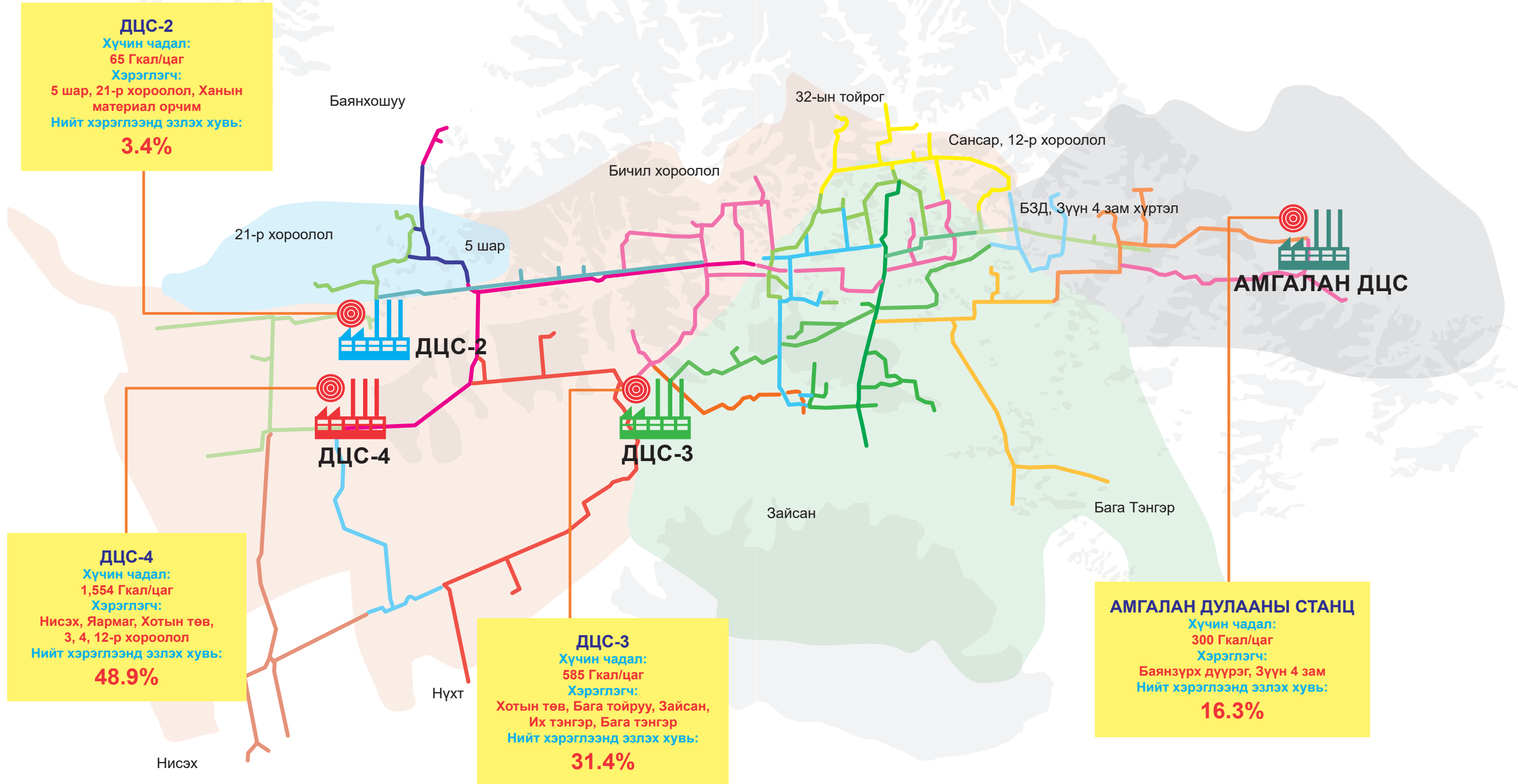
Зураг 9.9. Улаанбаатар хотын төвлөрсөн дулаан хангамжийн хамрах хүрээ
